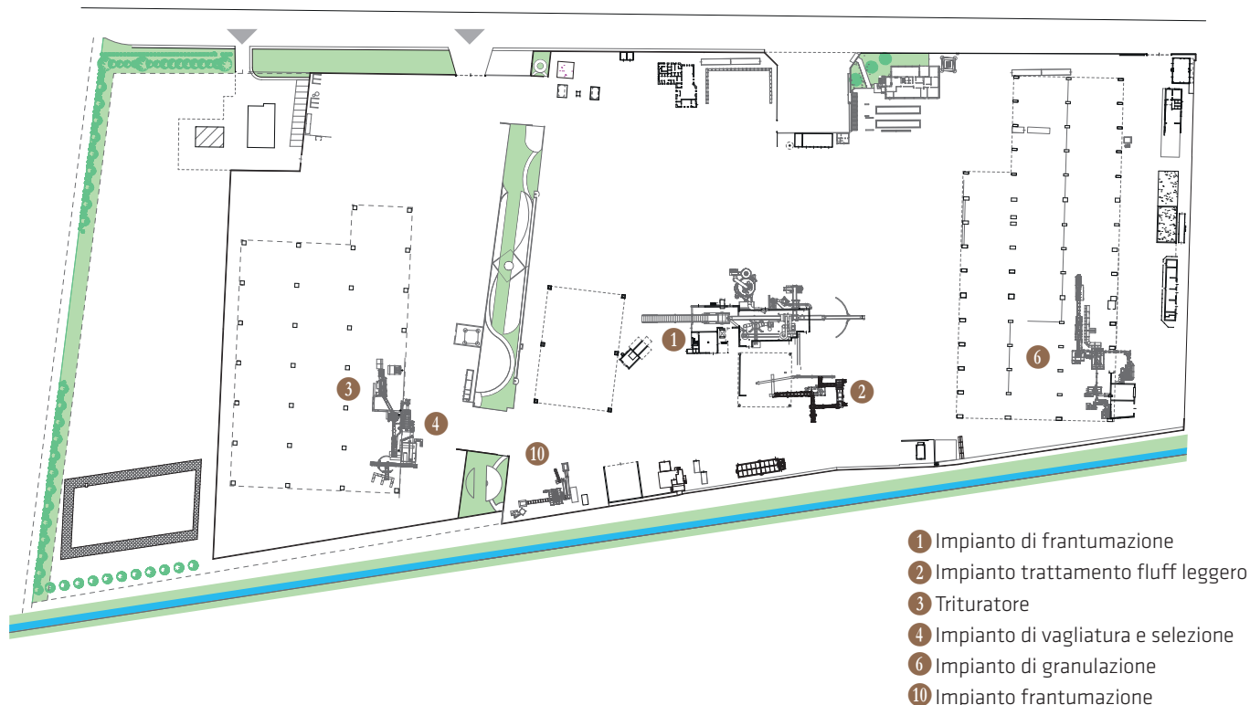
Fig. 2 Planimetria dell'impianto con l'indicazione dei numeri delle Linee - Scala 1:2500
